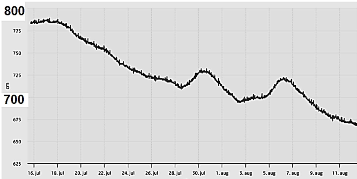
Figuur 2: Waterpeil Nijmegen haven na hoogwater medio juli 2024. Geregistreeerde waterhoogten boven NAP (Bron: Waterinfo.nl)
